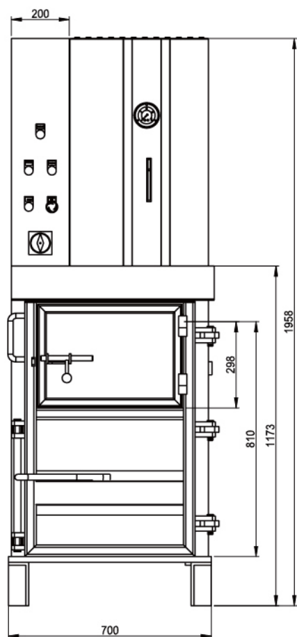
Diagram(Model XTY-50LA6545)
